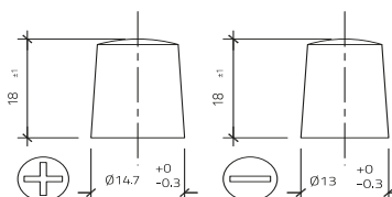
Polausführung 3
