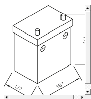
Maße
