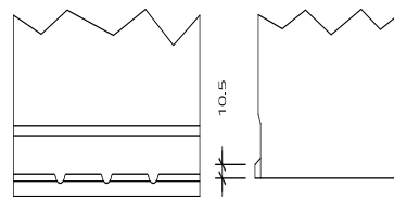
Bodenleiste B01
