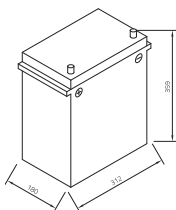
Maße
