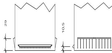
Bodenleiste B07
