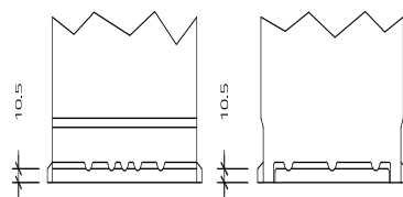
Bodenleiste B13
